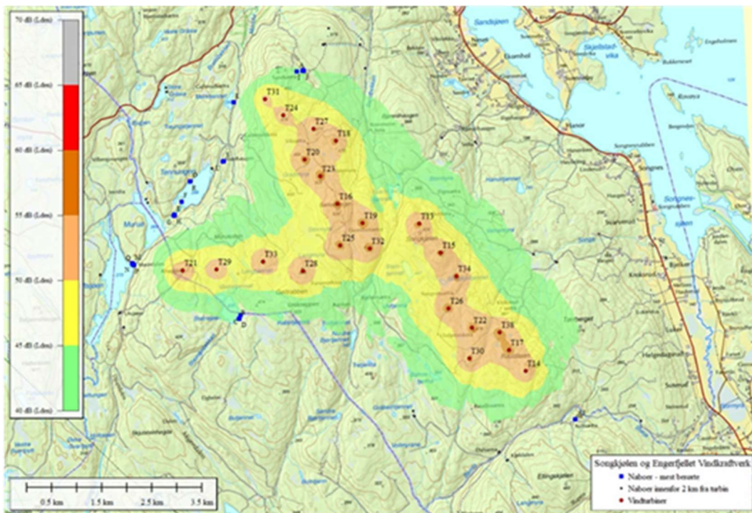
FIGUR 22 – STØYSONEKART FOR SONGKJØLEN BASERT PÅ BEREGET STØYNIVÅ ( L_{DEN} ) FOR REAL CASE (BEREGNING BASERT PÅ FAKTISK VINDFORHOLD)
